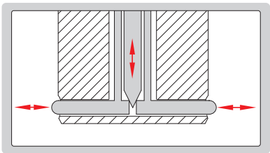
测量原理
